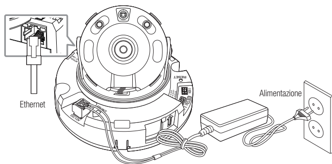
<QND-7012R/7022R/7032R>
