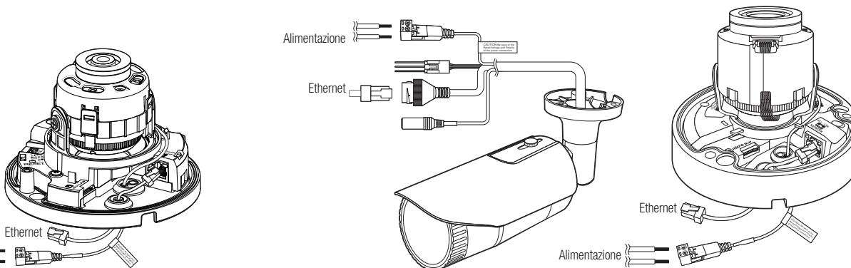
<QNV-6014R/7012R/7022R/7032R>
